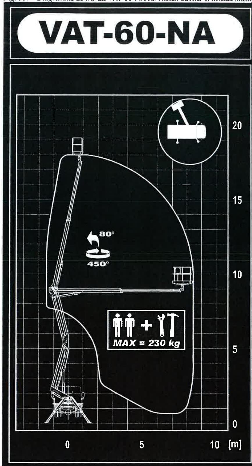
Fig. 13. Diagramme de travail VAT-60-NA sur Nissan Cabstar et Renault Maxity
