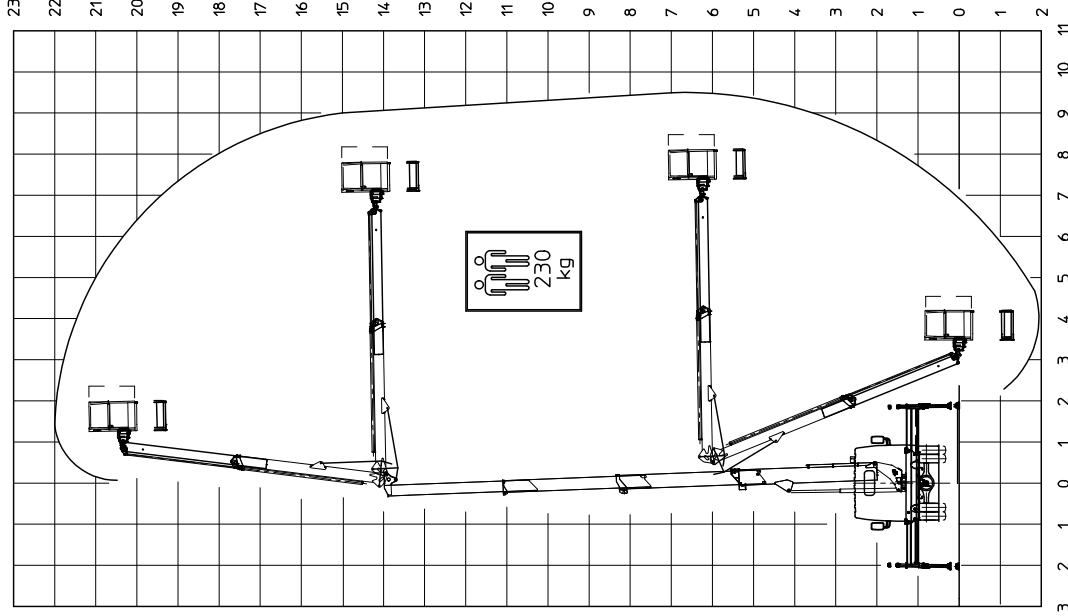
TRAVERSE ESTESE - OUTRIGGER OUT
